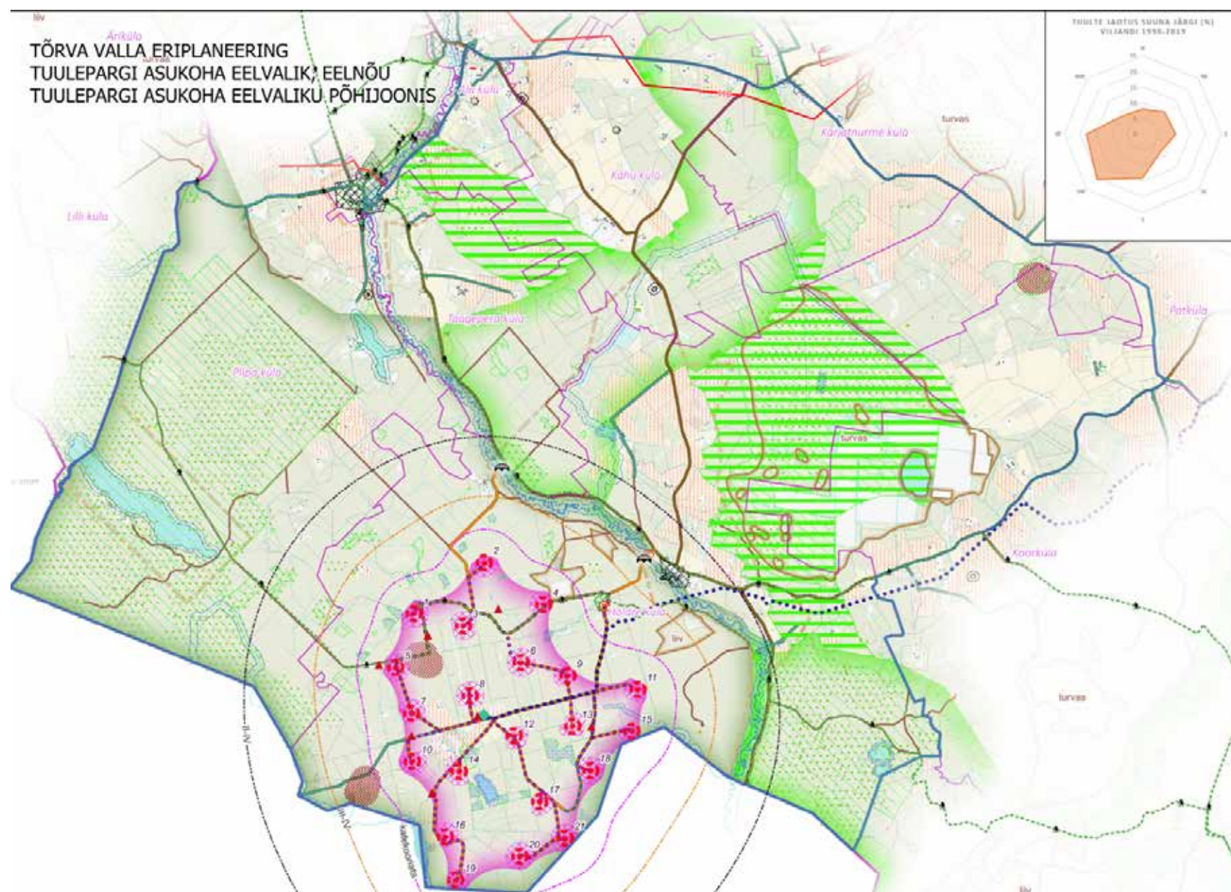
Kokku on planeeritud 21 tuulikut. Joonise koostaja AB Artes Terrae OÜ.
